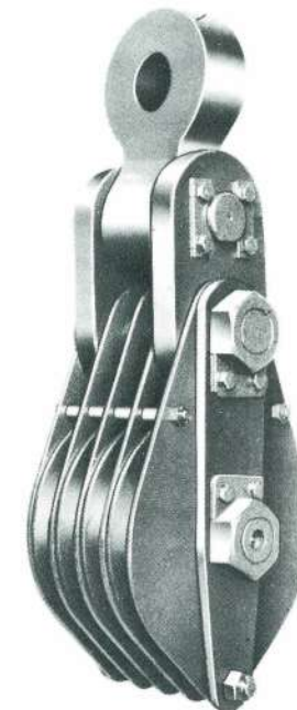
3. 40-ton Block with 4 Sheaves and Eye Block 目付ブロック
