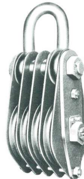
5. 30-ton Block with 4 Sheaves and Shackle シャクル式ブロック
